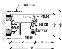
JAMB 5-1
