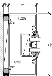
WALL JAMB
