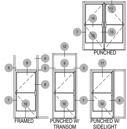
DOOR JAMB @OFFSET HUNG
