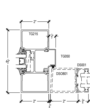
DOOR JAMB @OFFSET HUNG
