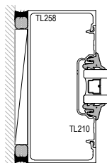
OPTIONAL JAMB
