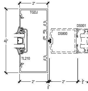
DOOR JAMB @CENTER HUNG
