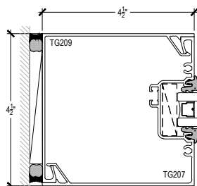
WALL JAMB ASSEMBLY
