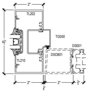
DOOR JAMB @OFFSET HUNG
