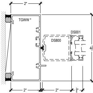
DOOR JAMB @CENTER HUNG
