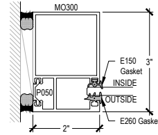
WALL JAMB
