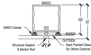
OPTIONAL SSG VERTICAL
